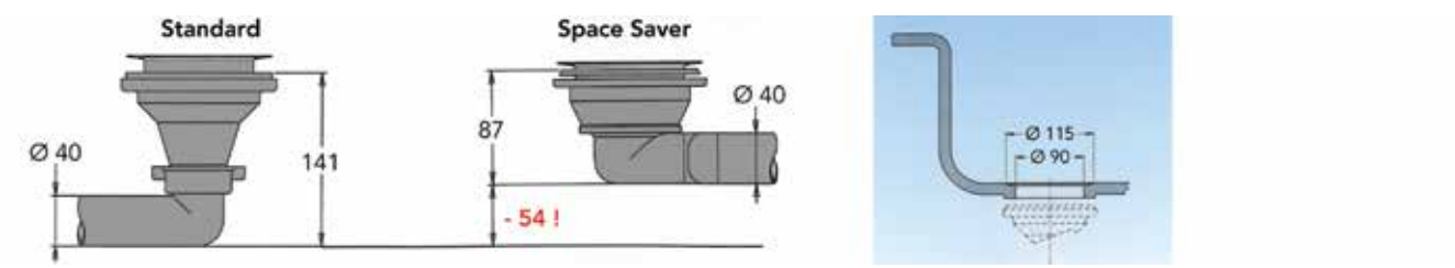
Crépine Space Saver sans trop plein
