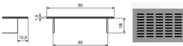
Grille d'aération avec hauteur 80 mm - petits trous ovales - petits trous ovales: 20 x 3 mm
