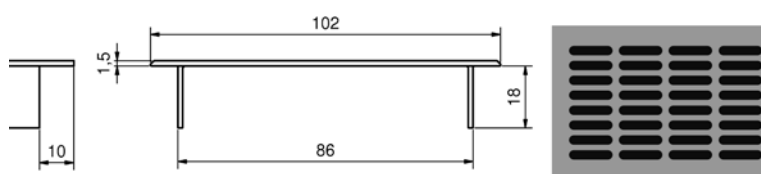
Grilles d'aération avec hauteur 102 mm - grands trous ovales - grands trous ovales: 30 x 6 mm
