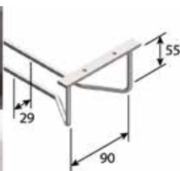
Support pour verres - montage au plafond
